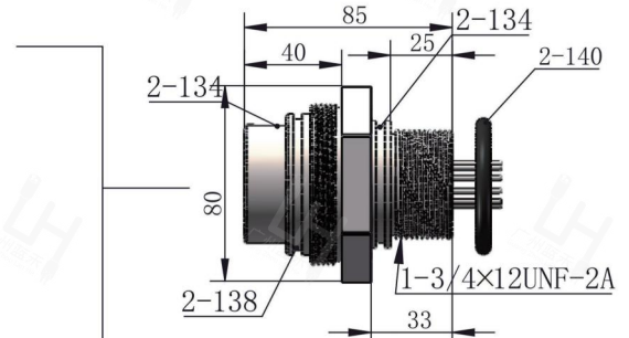
MSSN-10-BCR
