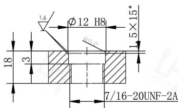
BCR安装孔位
