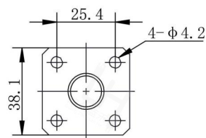
FCR安装孔位
