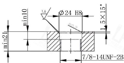
BCR安装孔位
